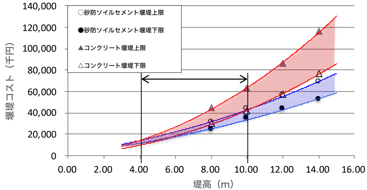
コスト比較
