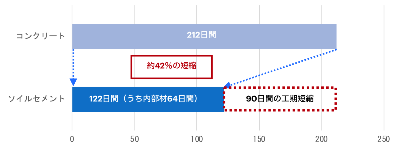
施工期間 (例)
